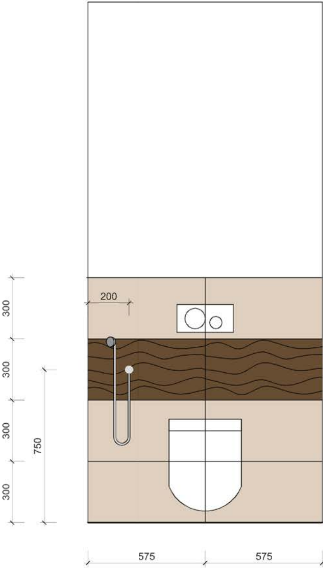
pohled 1
