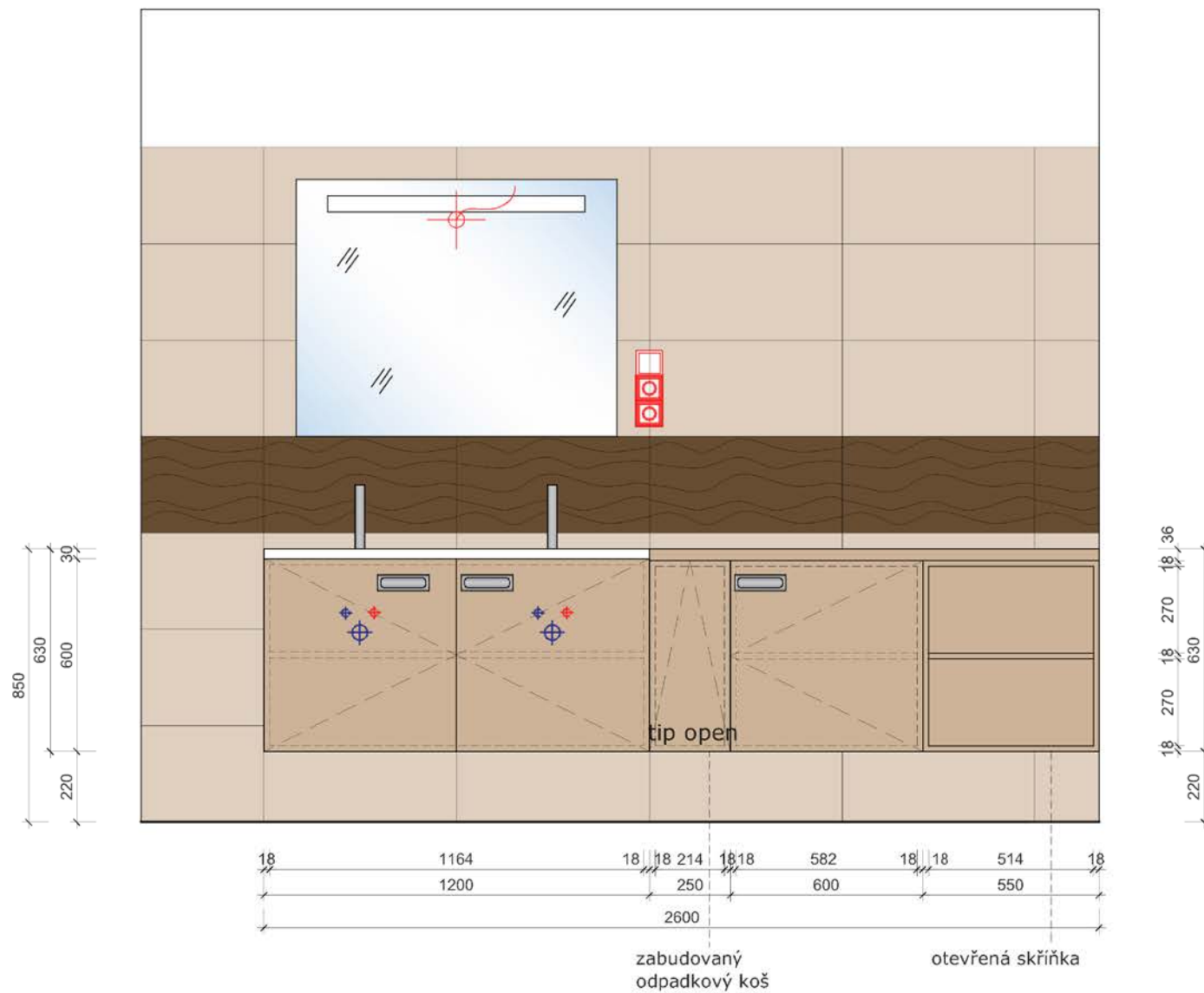
pohled 1
