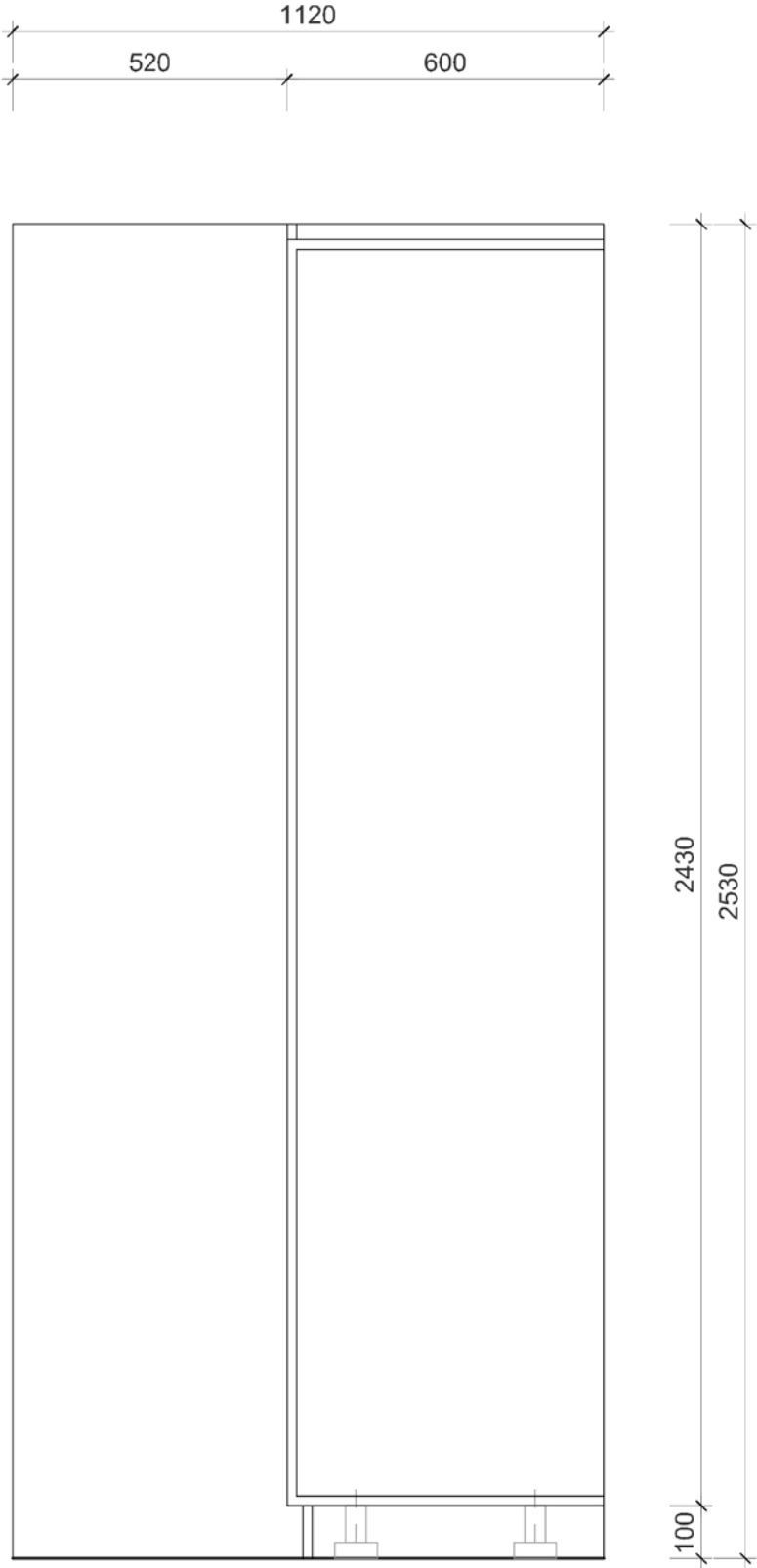
pohled 2
