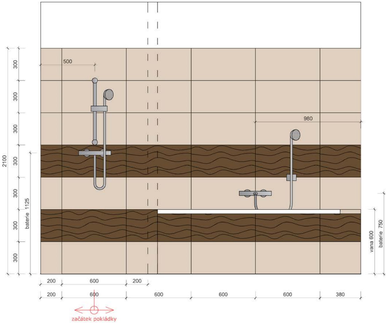
pohled 3
