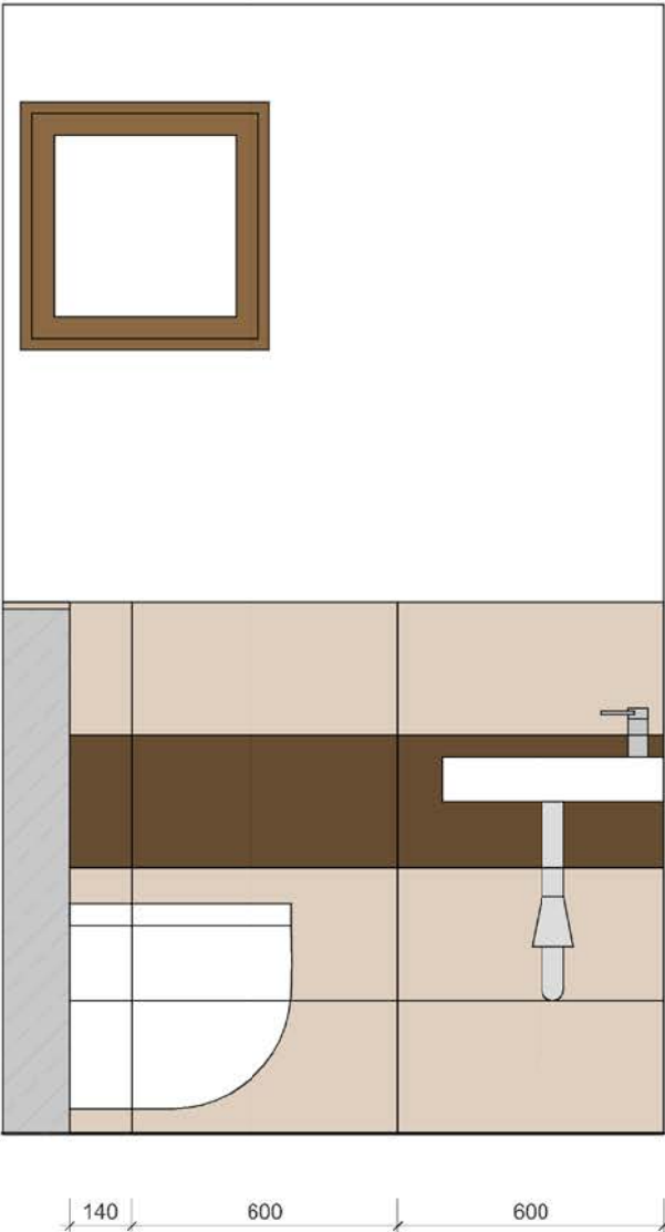
pohled 2
