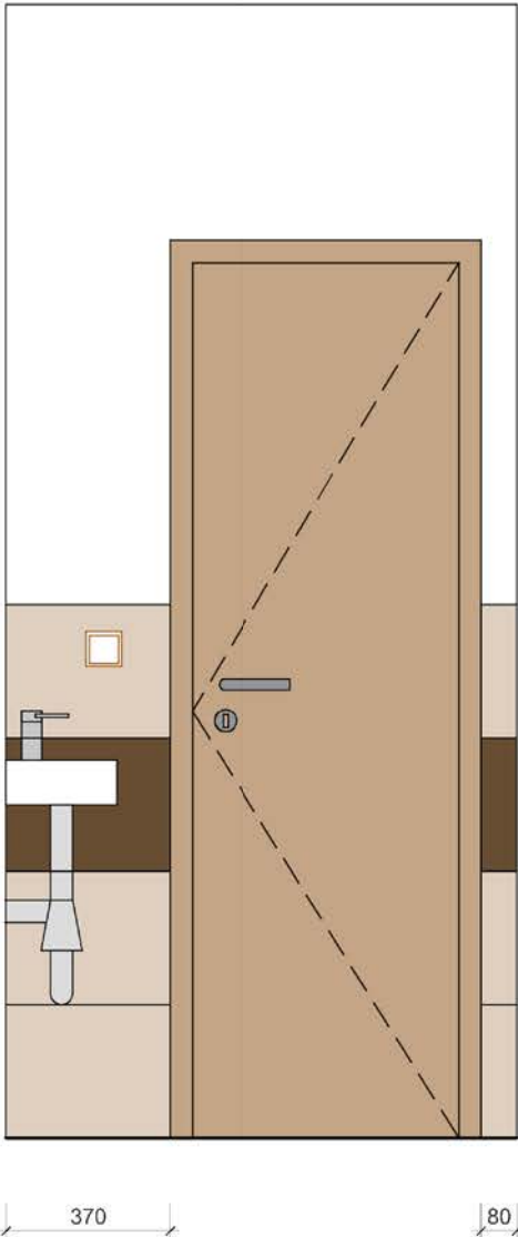
pohled 3
