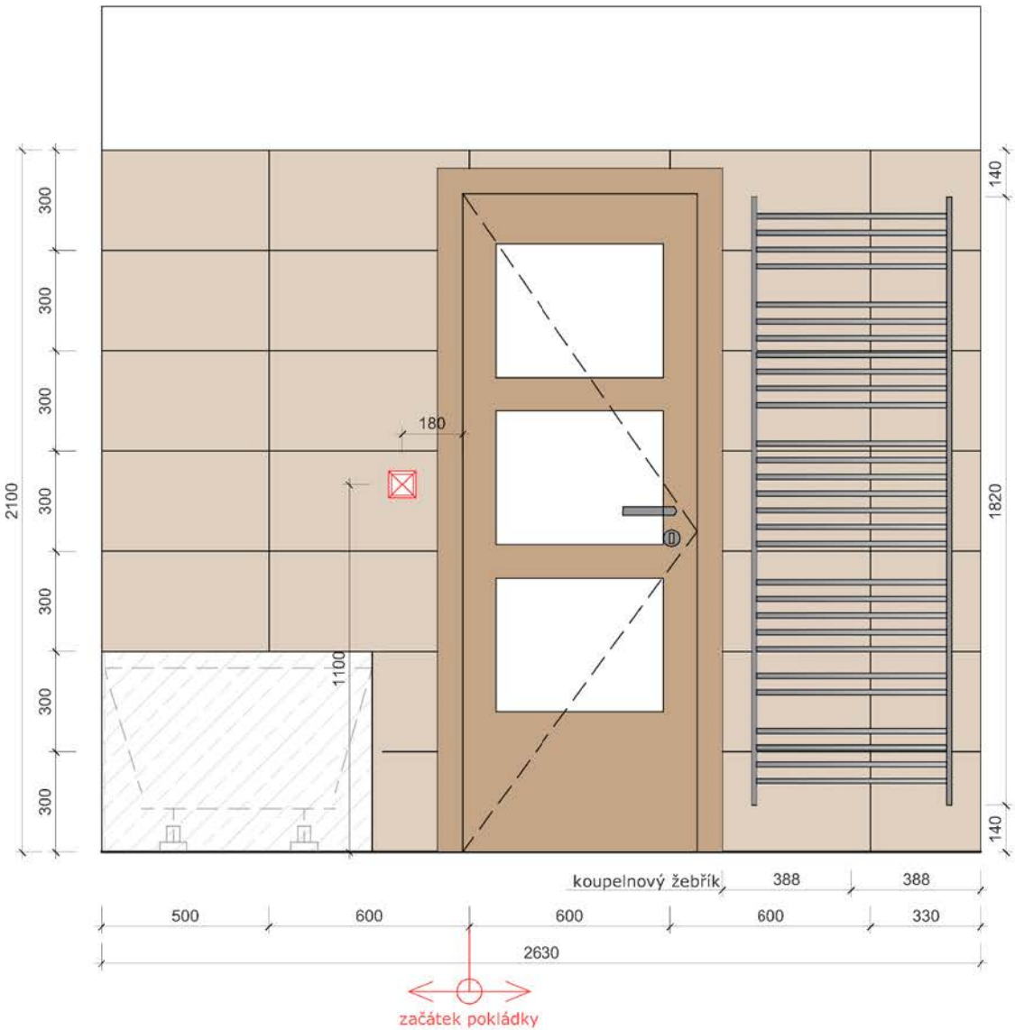
pohled 4
