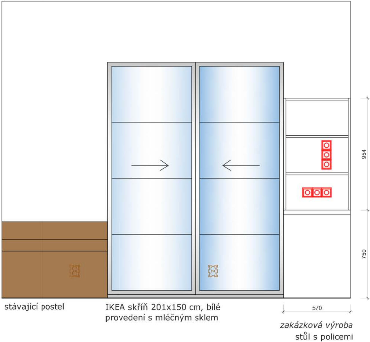
pohled 2
