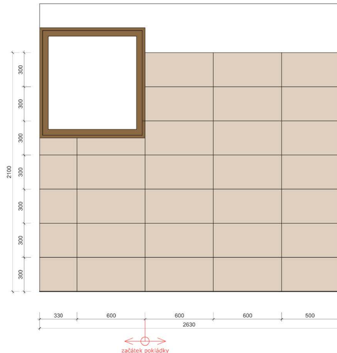
pohled 2
