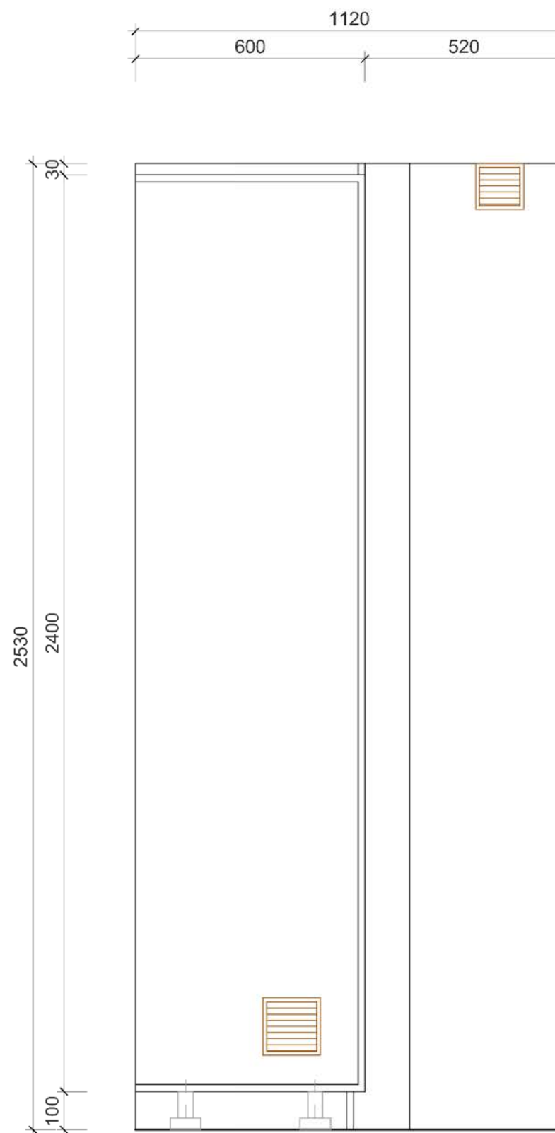
pohled 4
