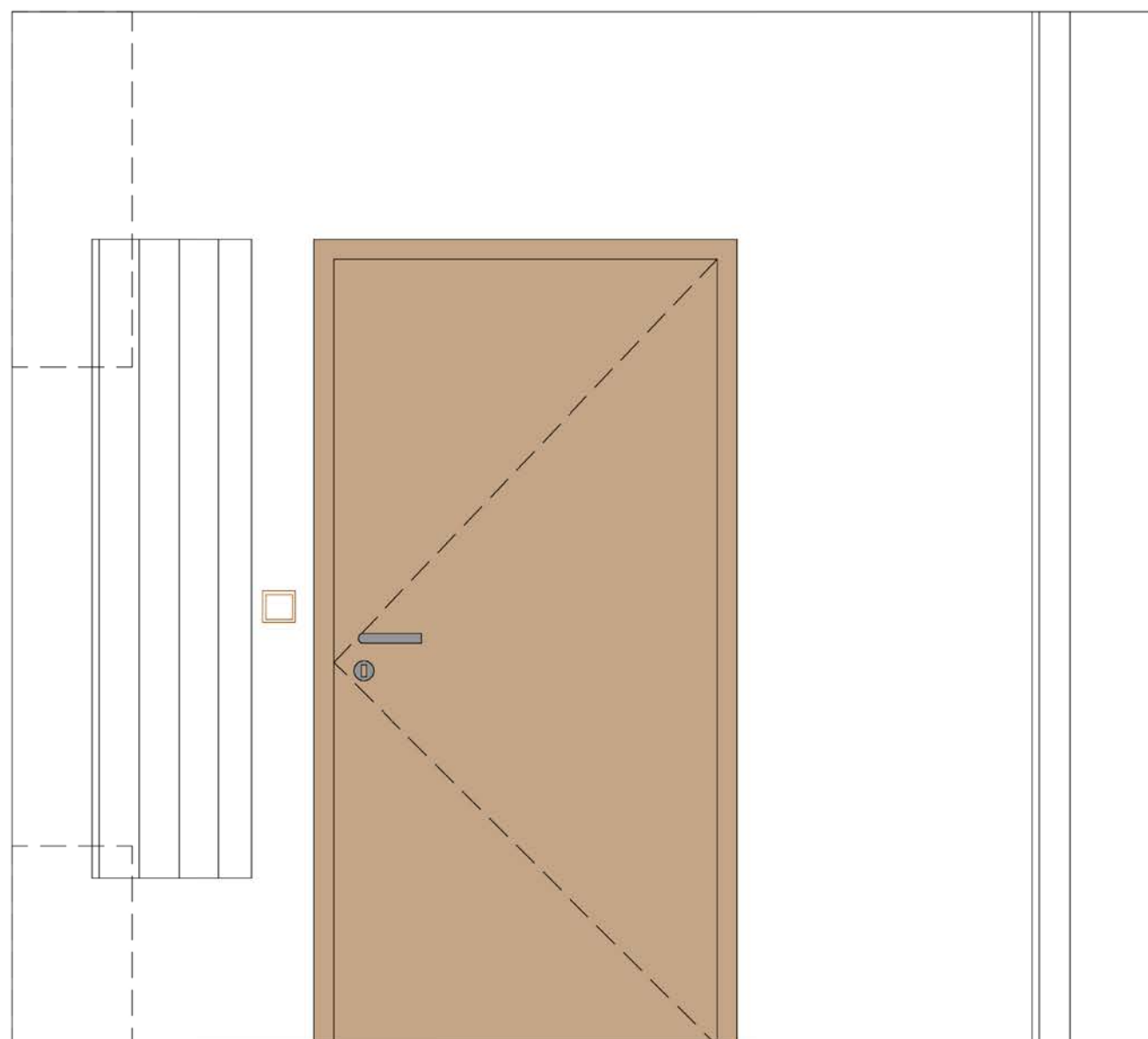
vertikální radiátor T20 40x160 cm, bílá barva
