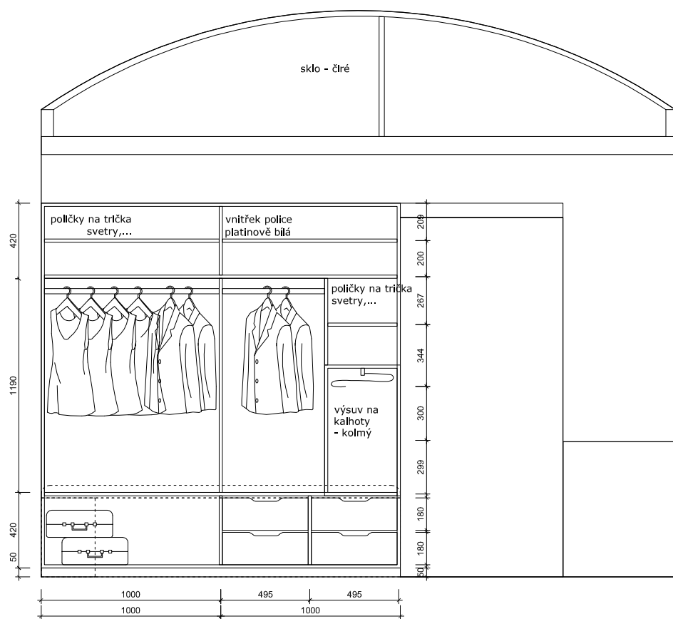
Pohled 7 - vnitřní rozložení stříně
