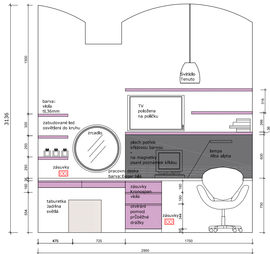
Pohled 7 - vnitřní rozložení stříně
