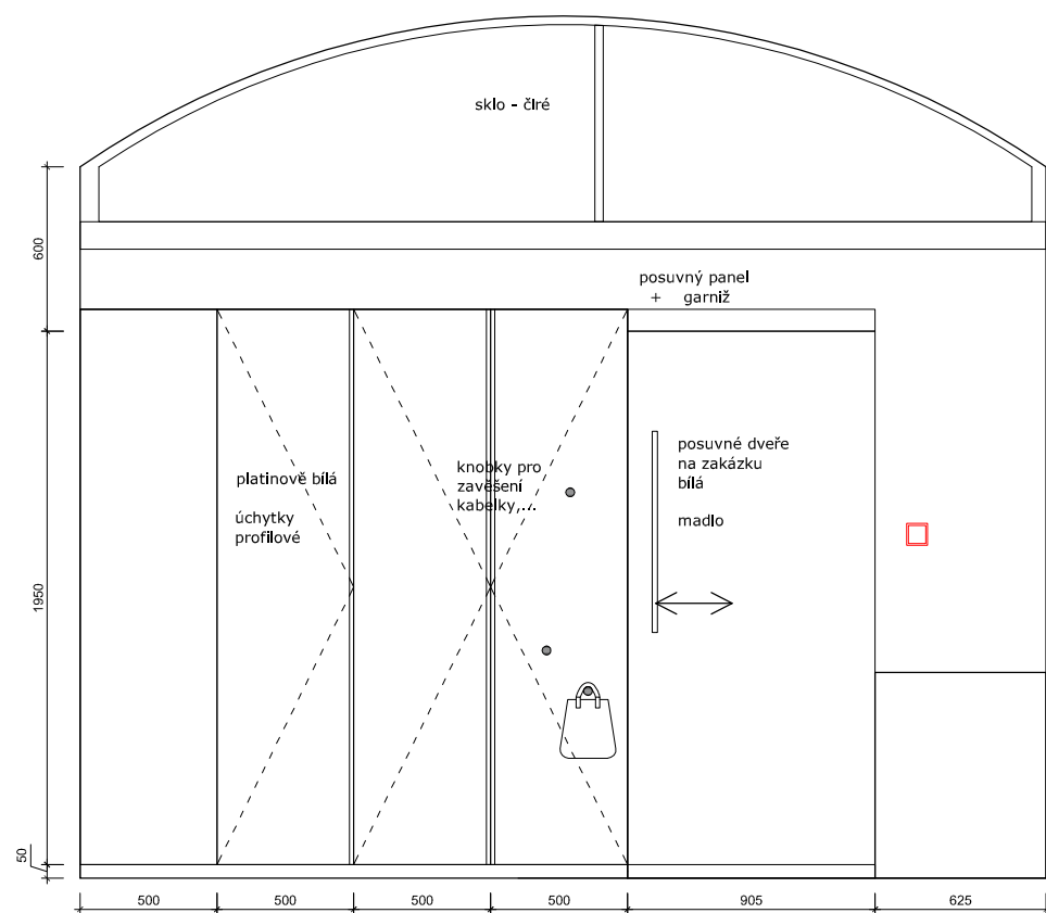
Pohled 7 - pohled na skříň
